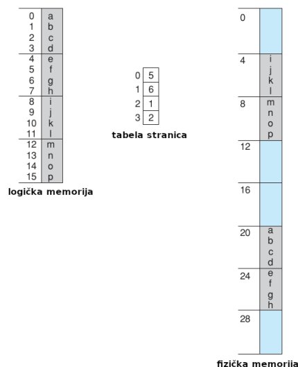
Slika 12: Primer jednostavne memorije sa stranicama
