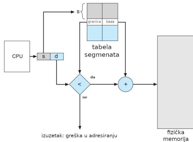
Slika 8: Hardver za segmentaciju
