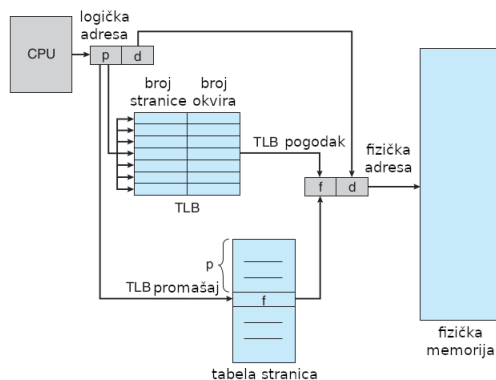
Slika 14: Hardver za straničenje sa TLB
