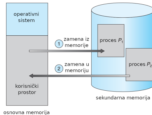
Slika 5: Zamena dva procesa korišćenjem diska kao sekundarne memorije
