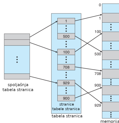
Slika 17: Tabela stranica sa dva nivoa
