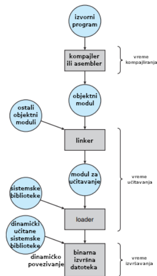
Slika 3: Pripremanje procesa za izvršavanje u nekoliko koraka
