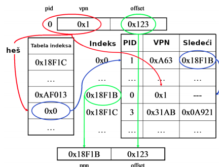
Slika 22: Heširana invertovana tabela stranica
