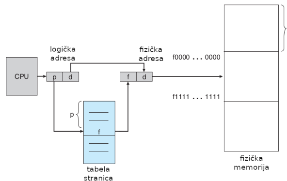
Slika 10: Hardver koji omogućava korišćenje stranica
