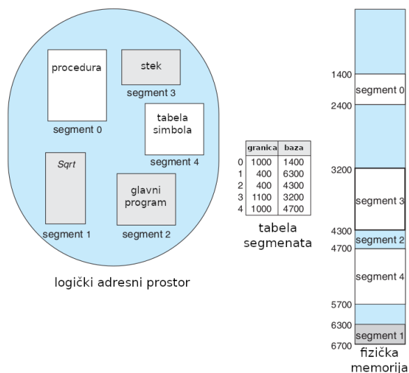
Slika 9: Primer segmentacije
