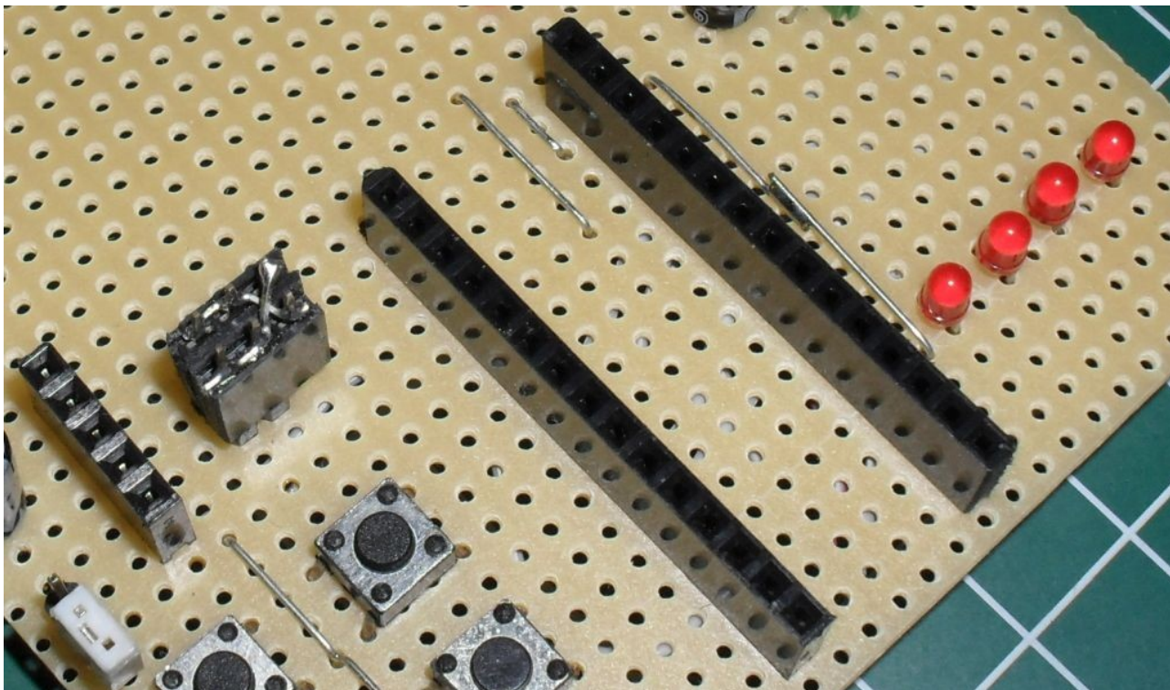
Slika 3 - Mesto za priključenje Arduinino Nano modula – u pitanju su dve jednorede ženske kontaktne letve koje odgovaraju kontaktnim letvama koje se standardno leme na Arduino Nano module. Na ovaj način modul se lako postavi i ukloni iz sistema. Jasno se vide i kratkospojnici koji su postavljeni sa gornje strane ploče, a krajevi su zalemljeni sa donje strane (provučeni su kroz rupu)
